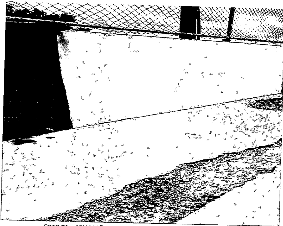
FOTO 21 – APLICAÇÃO DE SELADOR ACRILICO – MURETA – FONTE: AUTOR
