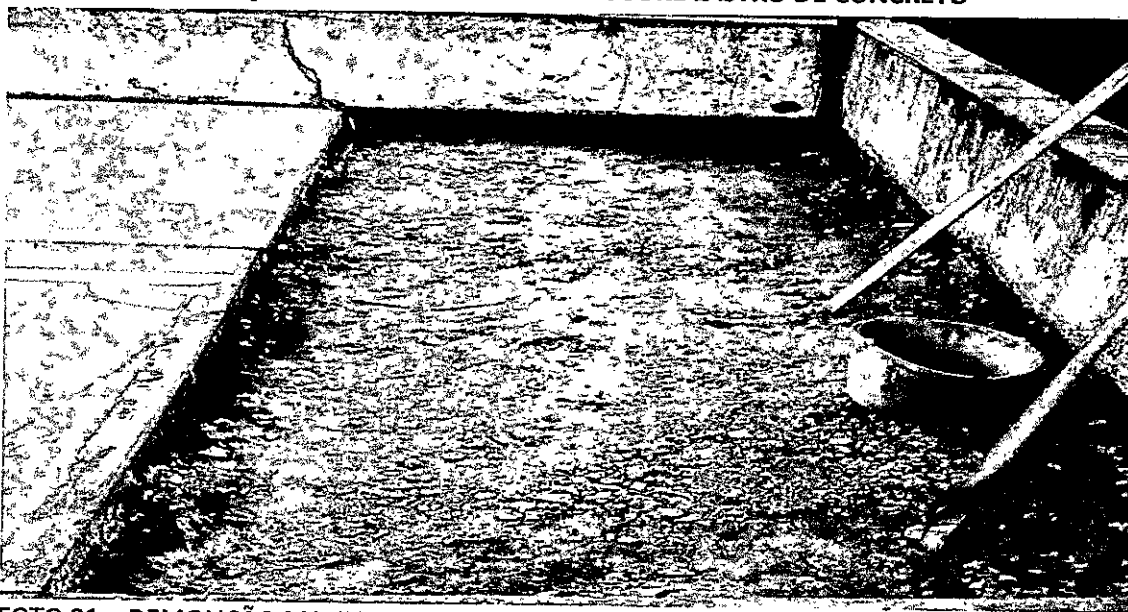
FOTO 01 - DEMOLIÇÃO MANUAL DE PISO - QUADRA - FONTE: AUTOR
