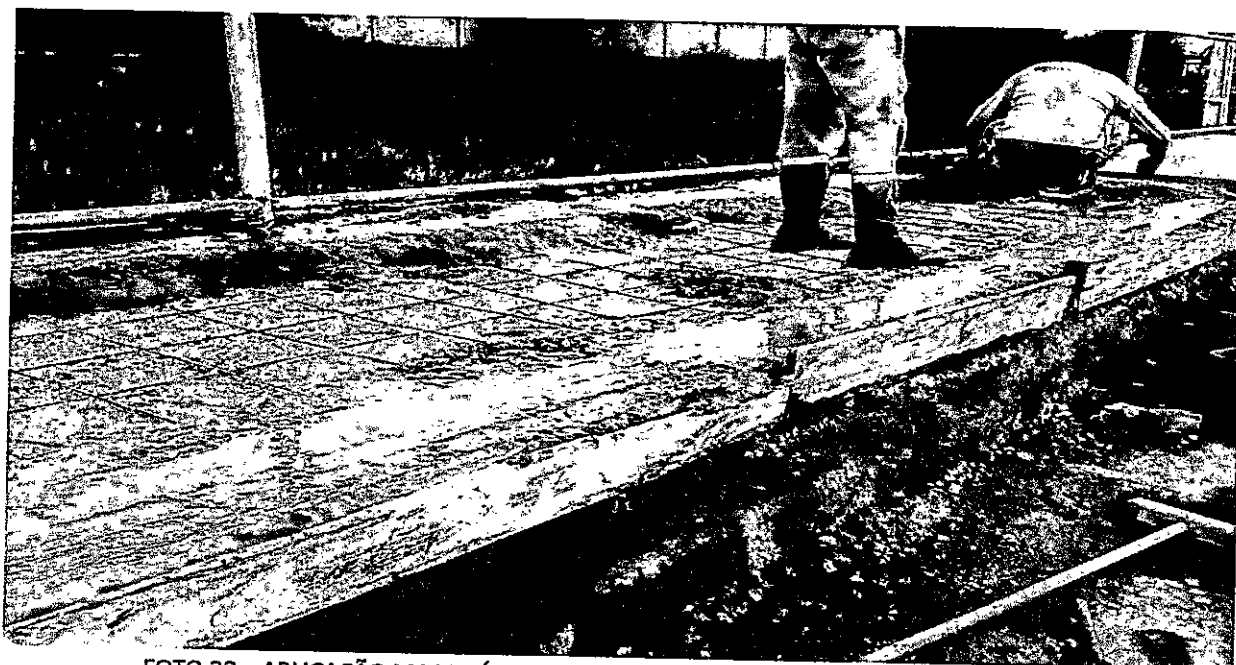
FOTO 22 – APLICAÇÃO MASSA ÚNICA – ASSENTO SUPERIOR – ARQUIBANCADA
